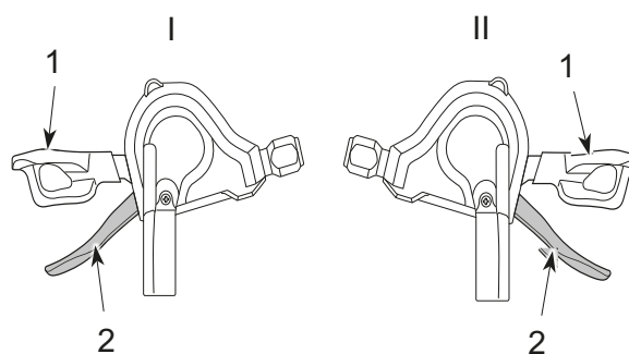
Illustration 85 : Manette de vitesse inférieure (1) et manette de vitesse supérieure (2) du changement de vitesse gauche (I) et droit (II)
