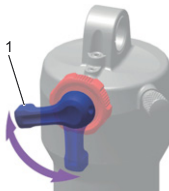
Illustration 84 : Régler la dureté de l'amortisseur de compression sur le levier (1) de l'amortisseur arrière
