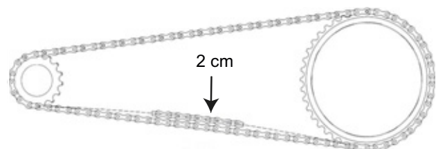
Illustration 87 : Contrôler la tension de la chaîne
