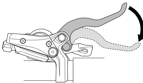
Obr. 54: Vzdálenost brzdové páky od řídicích
