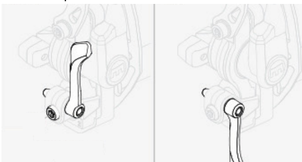
Obr. 10: Blokovací páka ráfkové brzdý, zavřená (1) a otevřená (2)
