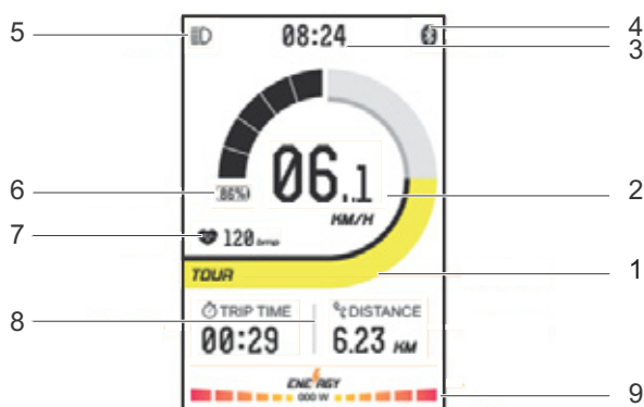
Obr. 20: Popis ukazatelů na displeji
