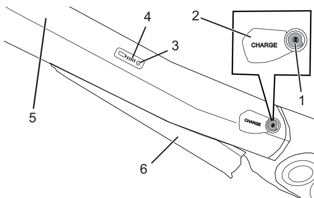
Obr. 15: Detail akumulátoru Evo 550
