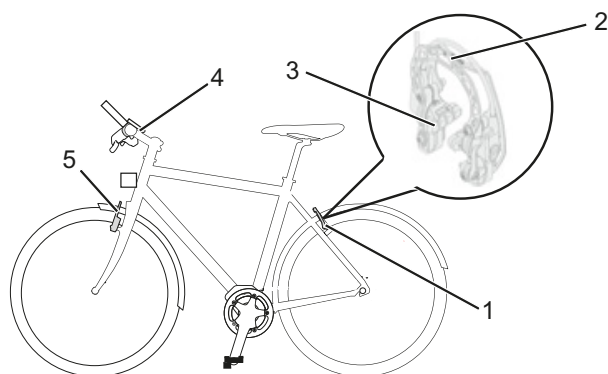
Obr. 9: Součásti ráfkové brzdý s detailem, příklad Magura HS22
