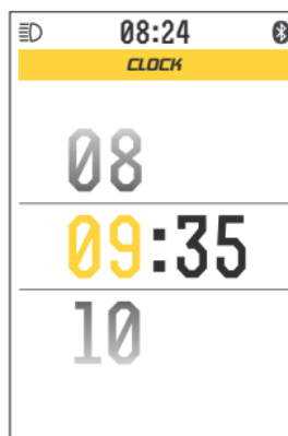
Obr. 74: Nastavit hodiny
