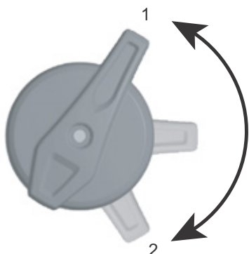
Obr. 76: Nastavovací šroub komprese FOX s polohami OTEVŘENÁ (1) a TVRDÁ (2)
