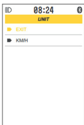
Obr. 69: Výběr jednotek
