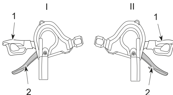
Obr. 92: Páčka pro řazení převodů dolů (1) a páčka pro řazení převodů nahoru (2) levého (I) a pravého (II) řazení
