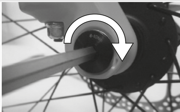
Obr. 29: Utáhněte osu
