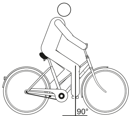
Obr. 53: Měření olovnicí od česky
