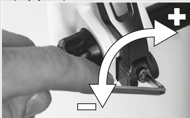
Obr. 96: Nastavení upínací síly rychloupínáku
