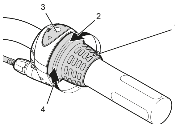
Obr. 93: Příklad řazení Shimano Nexus: Otočné řazení (1) vícerychlostního náboje s ukazatelem (3), se šipkou ukazující řazení nahoru (2) a řazení dolů (4)
