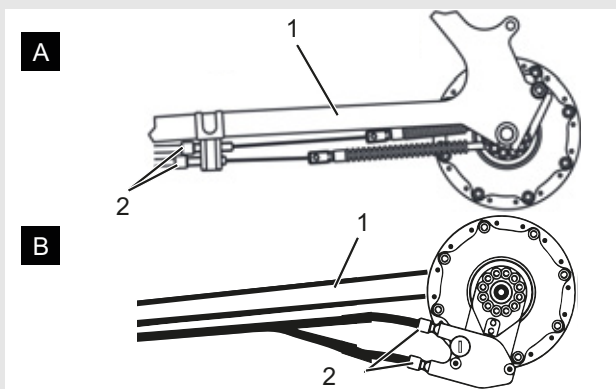
Obr.98: Nastavovací pouzdra (2) řazení převodů ve dvou alternativních provedeních (A, resp. B) s ovládáním dvěma lanky na zadní rámové stavbě (1)
