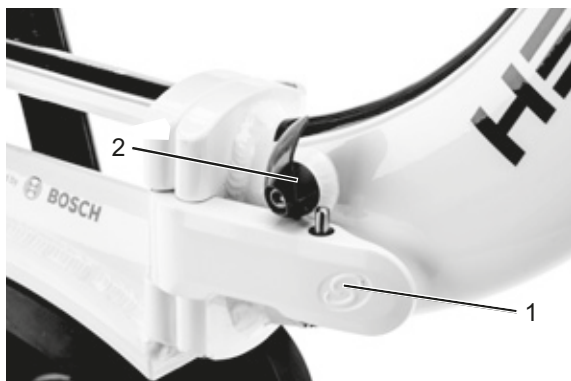
Obr. 73: Rám, s uzavřenou upínací pákou (1) a otevřenou pojistnou pákou (2)
