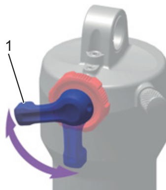
Obr. 91: Nastavení tvrdosti tlumiče komprese pákou (1) tlumiče zadního odpružení
