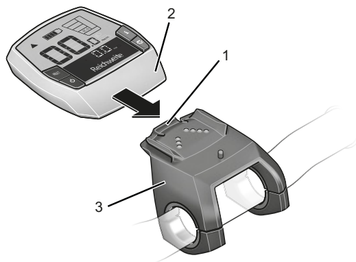
Obr. 82: Displej (2) přes aretaci displeje (1) posuňte až k dorazu držáku (3)
