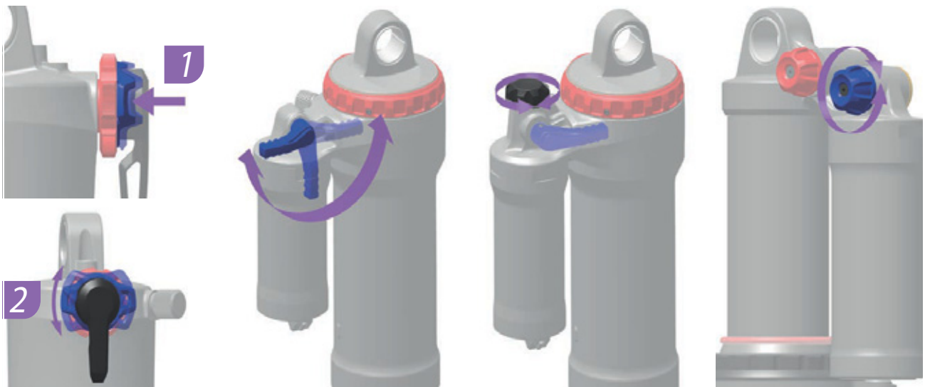
Figur 234: Tryktrins-indstillingsanordningens (blå) placering og form afhænger af den pågældende model
