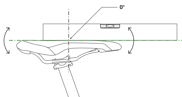
Figur 112: Vandret sadelhældning med 0° hældning i sadelmidten
