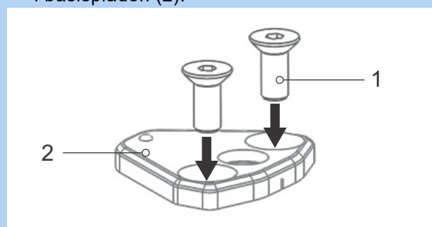
Figur 87: Indsætning af skruerne med undersænket hoved i basispladen
