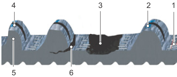
Figur 182: Tegn på slitage på en rem
