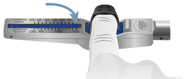
Figur 186: Pegefinger i kontrollære
