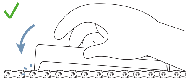
Figur 180: Målelæren passer ikke
