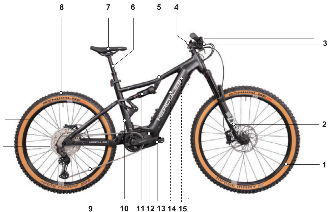
Figur 3: Elcykel set fra højre, eksempel HERCULES NOS FS 1.1
