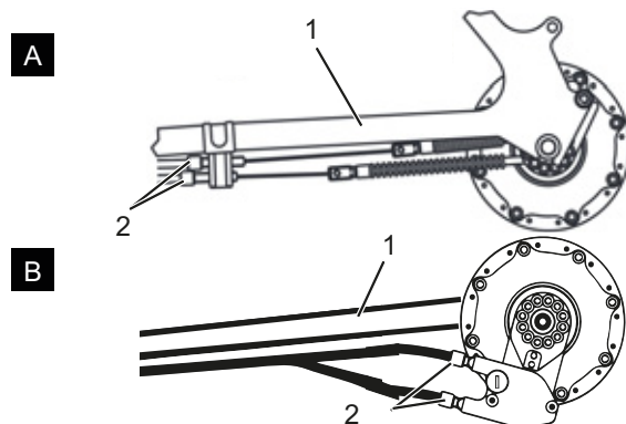
Figur 197: Slutmuffer (2) på to alternative udførelser (A og B) af et gearskifte med to kabler på baggafflen (1)
