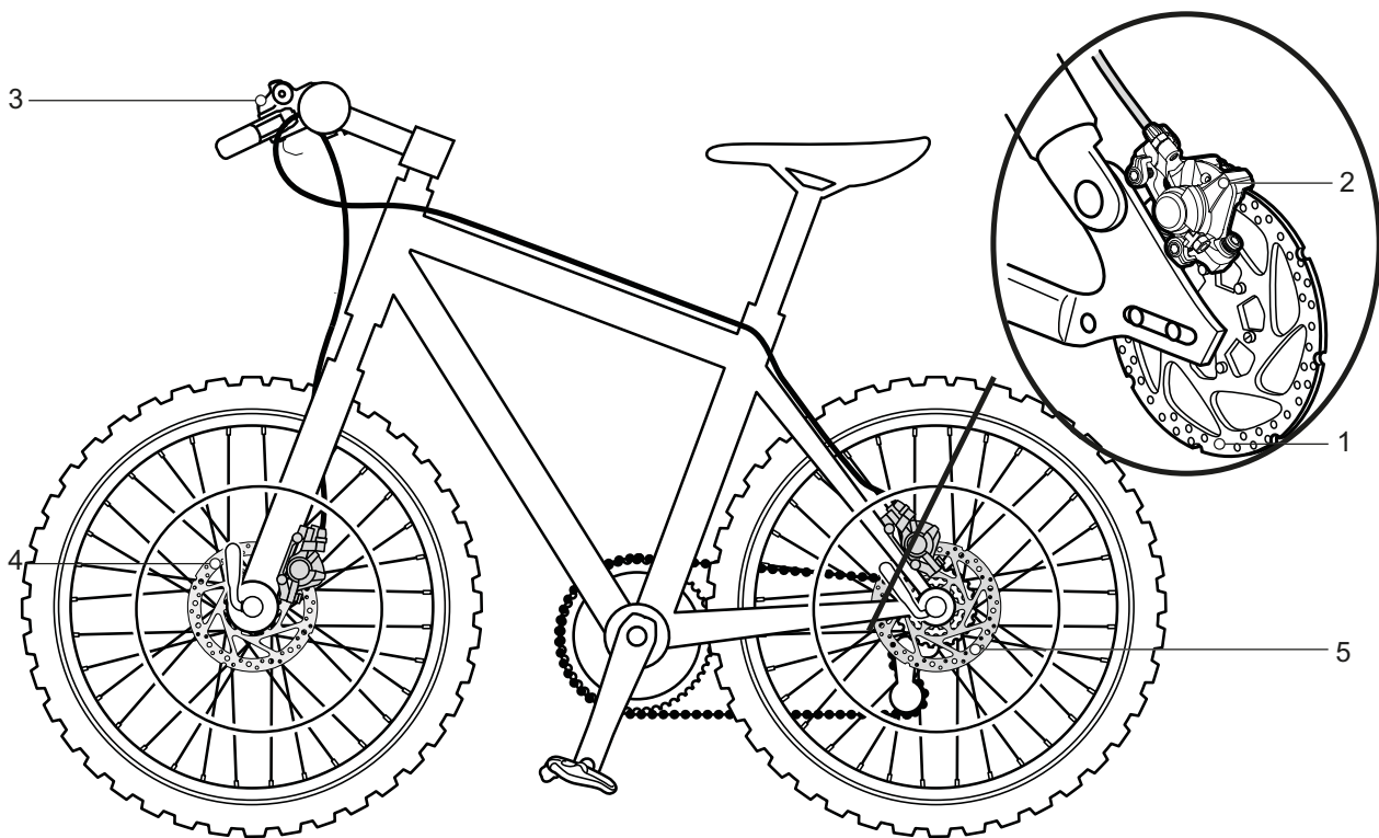
Figur 33: Bremsesystem med skivebremse, eksempel
