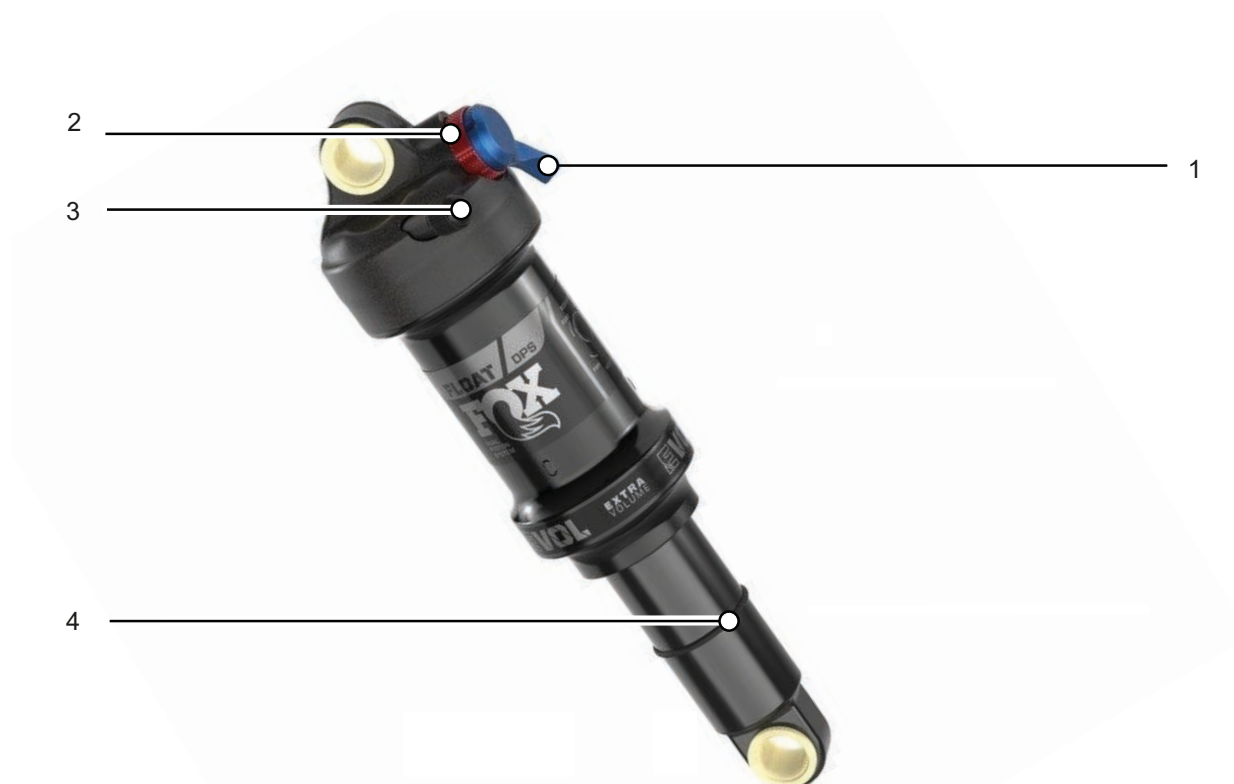
Figur 21: Eksempel med Monarch RL
