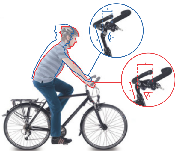
Figur 120: Position for citybike (blå) og trekkingcykel (rød) med vinkelændring
