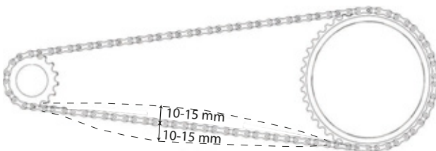
Figur 172: Eksempel på kontrol af kædestramning: 5 mm opad, 10 mm nedad = 15 mm afvigelse
