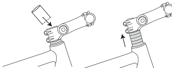
Figur 118: Forhøjning af Ahead-frempind ved at montere afstandsringe (spacers)
