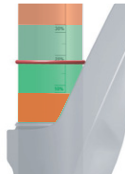
Rysunek 58: Zalecany zakres parametru SAG (zielony) i zakazany zakres parametru AG
