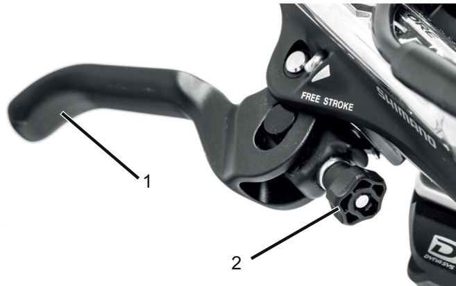
Illustration 20 : Levier de frein (1) avec vis moletée (2)
