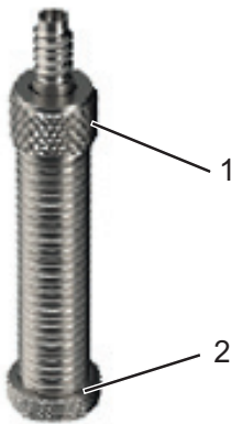
Illustration 25 : Valve Dunlop avec écrou-raccord (1) et écrou de jante (2)
