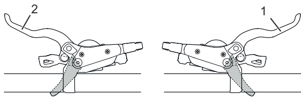
Abbildung 59: Bremshebel hinten (1) und vorne (2), Beispiel Shimano Bremse
