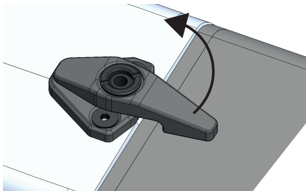
Abbildung 45: Sicherheitshebel öffnen
