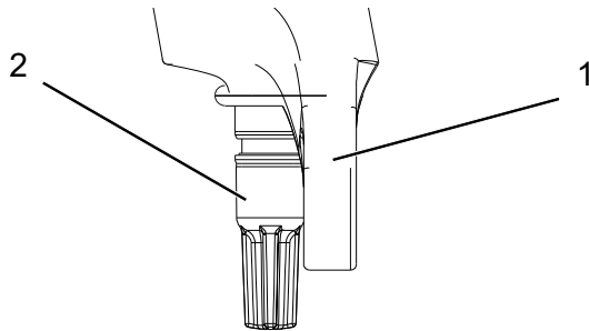
Abbildung 67: Suntour-Zugstufen-Schraube (2), Gabel (1)
