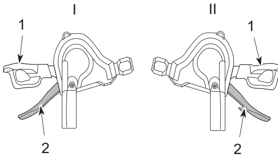
Abbildung 63: Runter-Schalthebel (1) und Hoch-Schalthebel (2) der linken (I) und rechten (II) Schaltung
