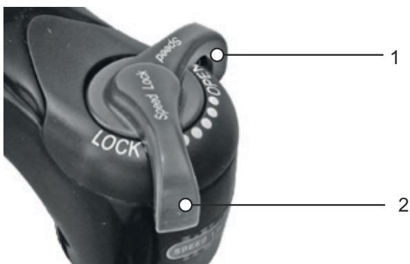
Abbildung 71: Suntour-Druckstufendämpfer in offener (1) und geschlossener (2) Position
